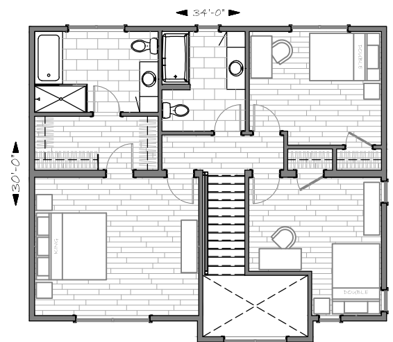
PLAN DU 2ème ÉTAGE
